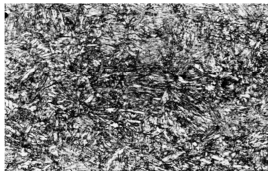
Bainitická štruktúra ocele
